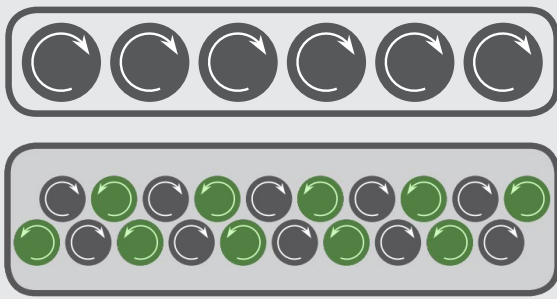
Gruppo spazzole tangenziali / sistema planetario Tangential brushes unit / planetary system Bürstenwalze tangential / planetarisch
