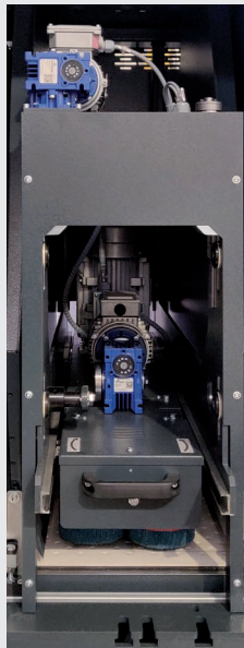
Gruppo spazzole tangenziali / sistema planetario Tangential brushes unit / planetary system Bürstenwalze tangential / planetarisch
